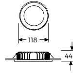
Tavan Kesim Ölçüsü: Ø 101
