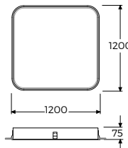
Tavan Kesim Ölçüsü: 1192X1192
