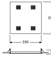
Tavan Kesim Ölçüsü: 580 x 580
