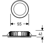
Tavan Kesim Ölçüsü: Ø 74
