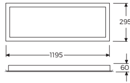
Tavan Kesim Ölçüsü: 280 x 1180
