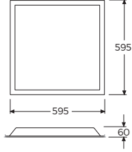
Tavan Kesim Ölçüsü: 580 x 580
