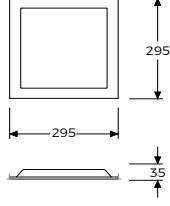
Tavan Kesim Ölçüsü: 280 x 280
