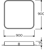
Tavan Kesim Ölçüsü: 892X892
