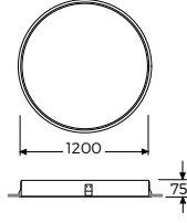
Tavan Kesim Ölçüsü: Ø 1192
