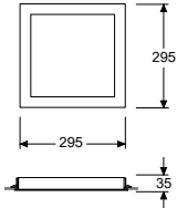
Tavan Kesim Ölçüsü: 280 x 280
