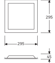
Tavan Kesim Ölçüsü: 280 x 280
