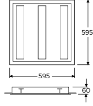
Tavan Kesim Ölçüsü: 580 x 580
