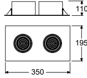
Tavan Kesim Ölçüsü: 170x315
