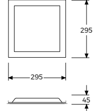
Tavan Kesim Ölçüsü: 280 x 280
