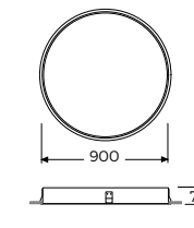
Tavan Kesim Ölçüsü: Ø 892
