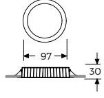
Tavan Kesim Ölçüsü: Ø 77
