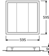
Tavan Kesim Ölçüsü: 580 x 580
