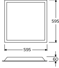
Tavan Kesim Ölçüsü: 580 x 580
