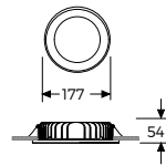
Tavan Kesim Ölçüsü: Ø 151
