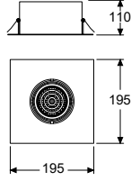
Tavan Kesim Ölçüsü: 170x170
