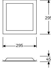
Tavan Kesim Ölçüsü: 280 x 280
