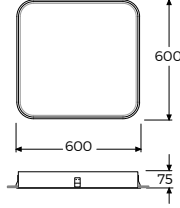
Tavan Kesim Ölçüsü: 592X592
